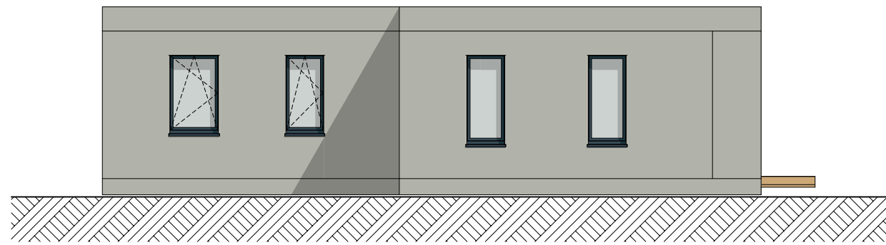
FACADE OUEST
